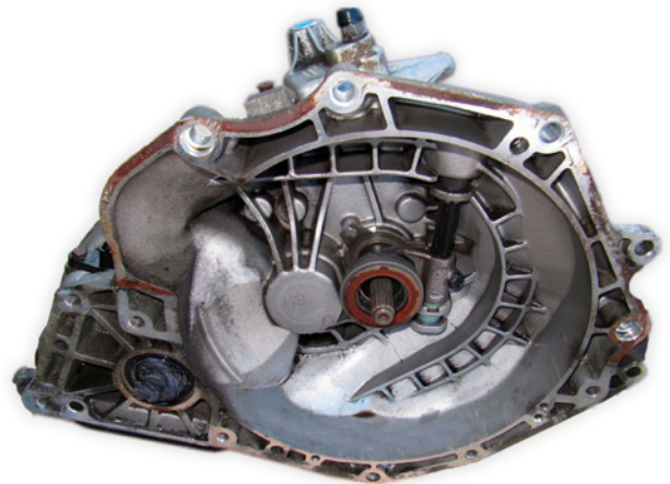
Bild 1: Bei Kupplungsreparaturen ist die Lagerung der Ausrückwelle zu prüfen
