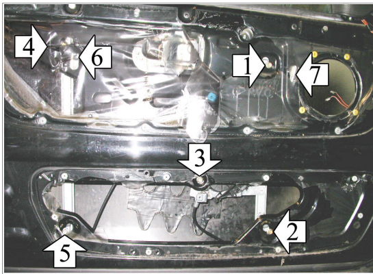
2 Doors - 2 Portes - 2_Türig - 2 Puertas - 2 Porte left door - portière gauche - linke tür - puerta lado izquierdo - porta lato sinistro
